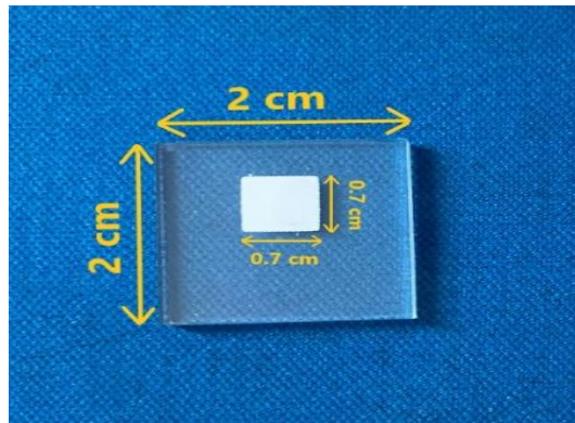
Şekil 6. \text{TiO}_2 nanopartiküllerinin FTO altlık üzerine kaplanması
