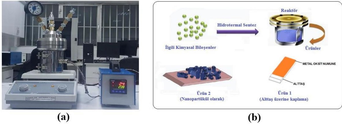
Şekil 5. Hidrotermal sentez düzeneği (a) ve ürün eldesi (b)
