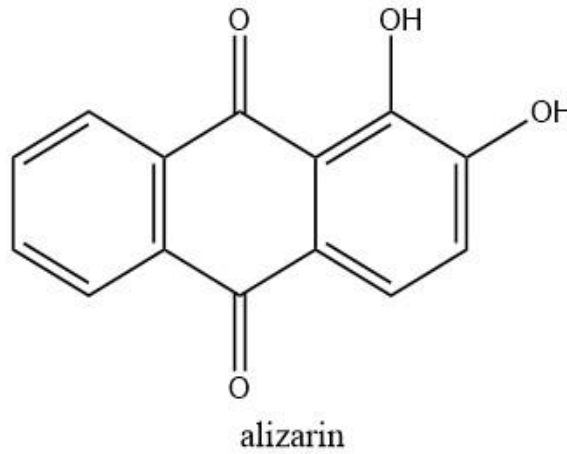
Şekil 7. Alizarinin kimyasal yapısı
