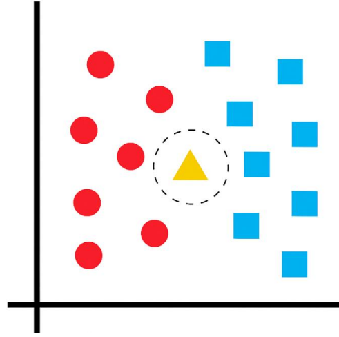
Şekil 3. K-En Yakın Komşu Algoritması İçin İki Sınıflı Örnek
