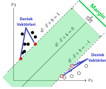
Şekil 4. İki Sınıfın SVM Hiper Düzlemi (Ayhan ve Erdoğan, 2014)
