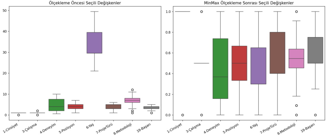
Şekil 9. Seçili Değişkenlerde MinMax Ölçekleme Öncesi ve Sonrası Dağılımı
