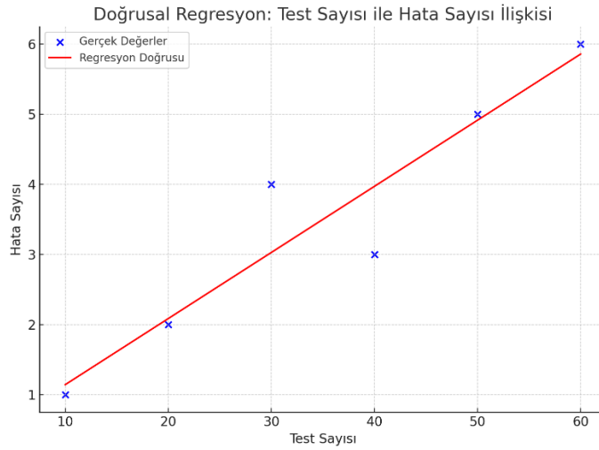
Şekil 2. Doğrusal Regresyon Modeli (James vd., 2021).
