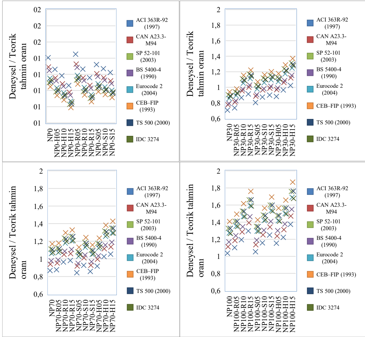
Şekil 18. Deneyisel ve teorik elastisite modülü değerlerinin oranı
