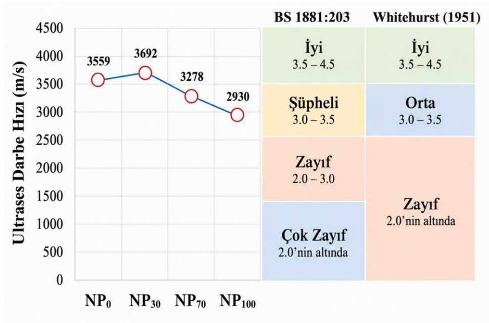
Şekil 27. UPV sonuçları.
