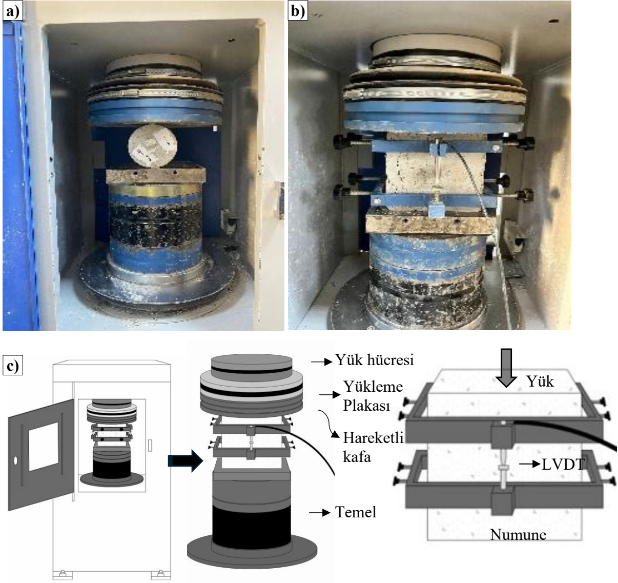
Şekil 12. Mekanik deney düzenekleri: a) yarmada çekme deneyi, b) basınç deneyi ve c) LVDT'ler kullanılarak gerçekleştirilen birim şekil değişirme ölçüm düzeneği.
