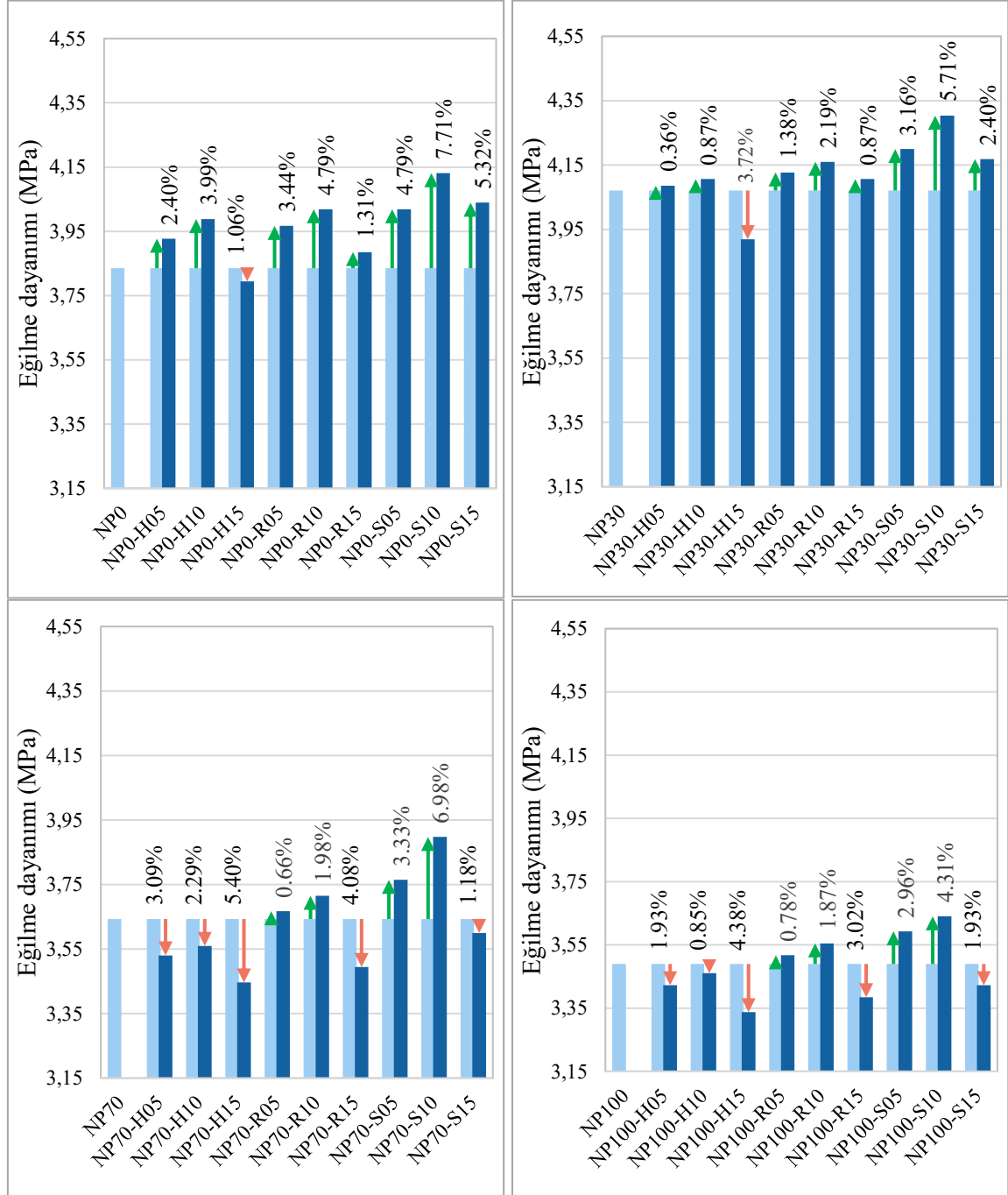
Şekil 32. Eğilme dayanımları
