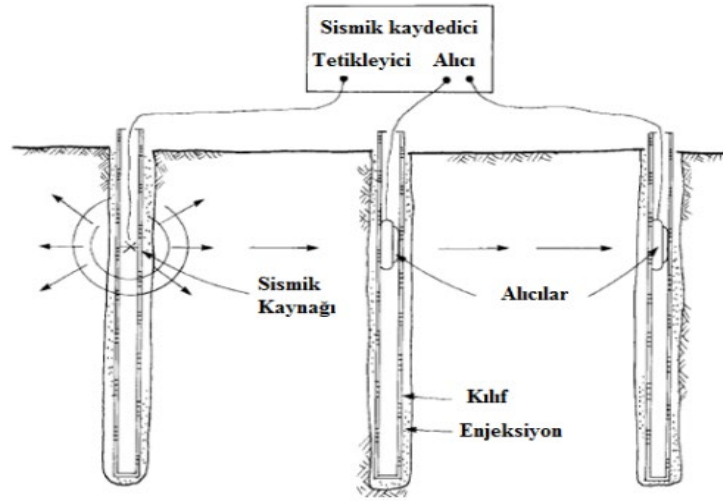
Şekil 2.16 Karşıt kuyu sismik deney düzeneginin şekil ile gösterimi (ASTM D 4428)
