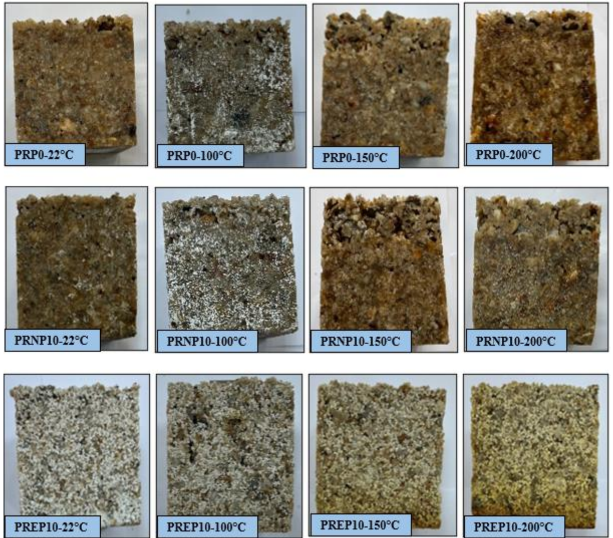
Şekil 27. Yüksek sıcaklık sonrası polyester reçineli polimer betonların görüntüleri
