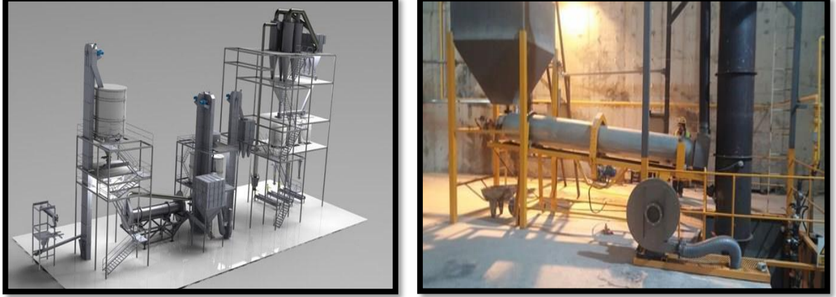
Şekil 11. Dikey ve yatay roket fırını (Başar, 2023; IPS Madencilik, 2025)
