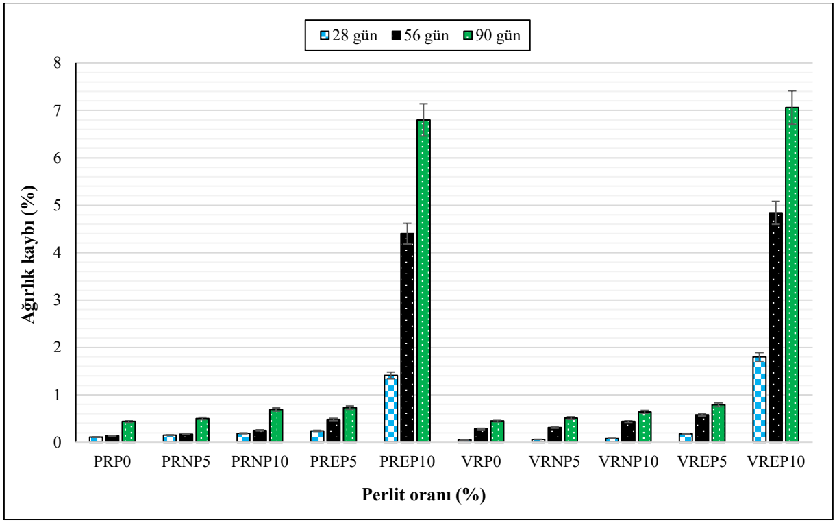
Şekil 22. Sülfat saldırısı sonrası polimer betonların ağırlık kaybı sonuçları
