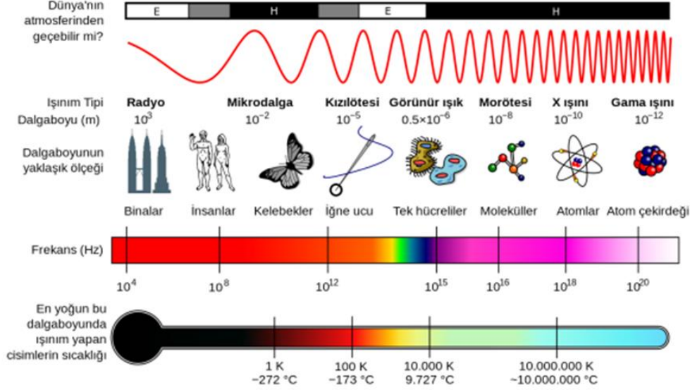
Şekil 1. Elektromanyetik Spektrum
