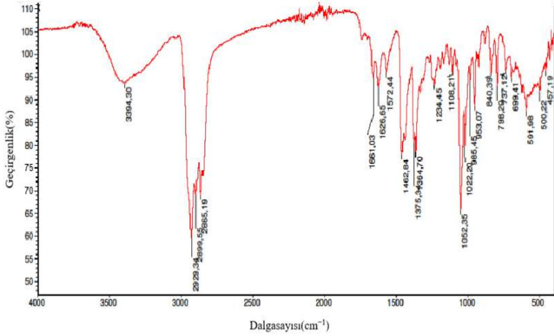
Şekil 4.7. Kolesterol-bilurabin karışık taşlarının FTIR spektrumu
