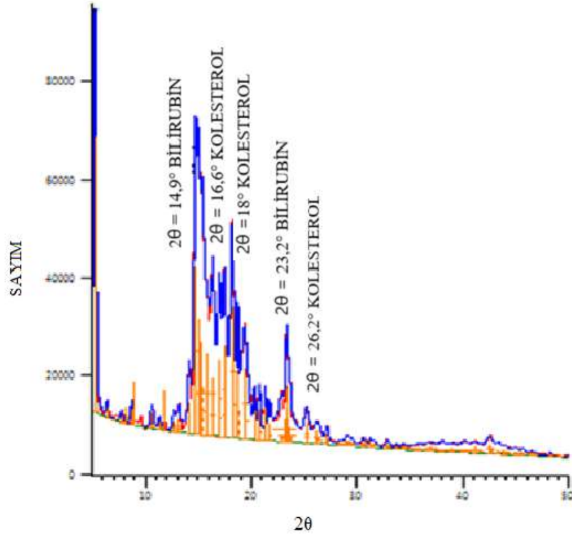
Şekil 4.14. Kolesterol-bilurabin karışık tipteki safra taşının XRD deseni
