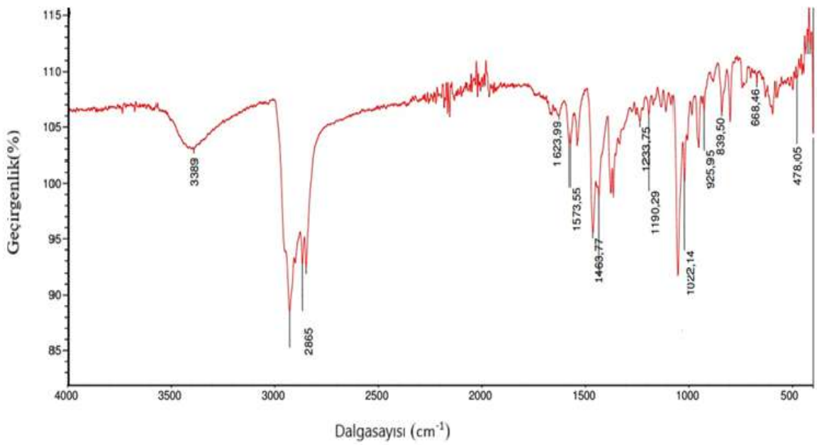
Şekil 4.6. Bilurabin taşlarının FTIR spektrumu
