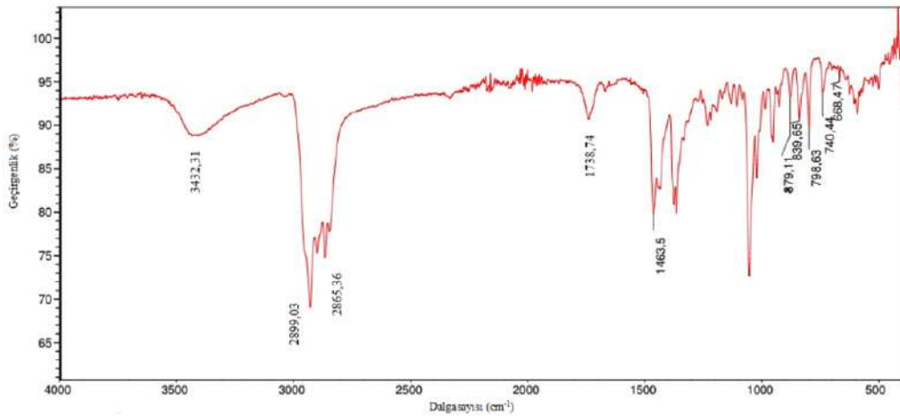
Şekil 4.4. Kalsiyum-karbonat taşlarının FTIR spektrumu
