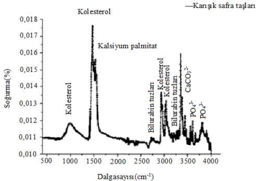
Şekil 4.10. Farklı safra taşı türlerinin tek bir FTIR spektrumu üzerinde gösterimi
