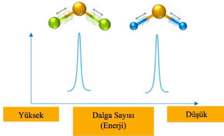
Şekil 3.2. Kızılötesi (IR) ışık moleküler titreşimleri başlatabilmekte olup gerekli enerji, bağların gücüne ve kütelere bağlıdır
