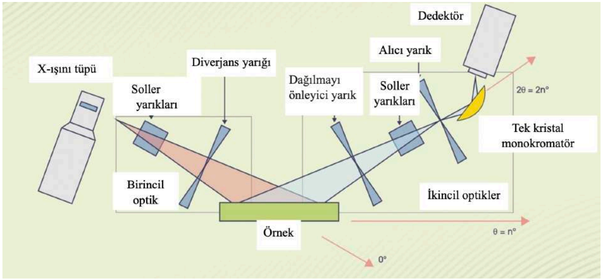
Şekil 3.7. Yaygın bir XRD enstrümantal düzeninin diyagramı
